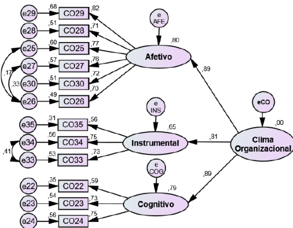
Figura 1 – Diagrama do modelo final do construto de segunda ordem: Clima Organizacional
