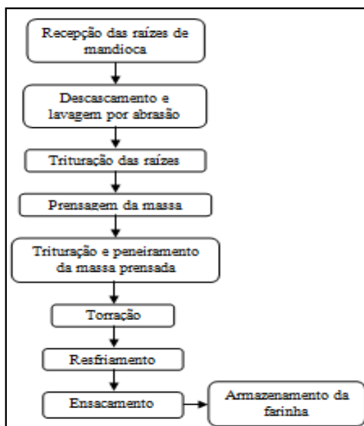
Figura 1. Fluxograma do processo, mecanizado, de beneficiamento de raízes de mandioca para obtenção de farinha de mesa, Sítio Chã do Jardim, Areia/PB.
