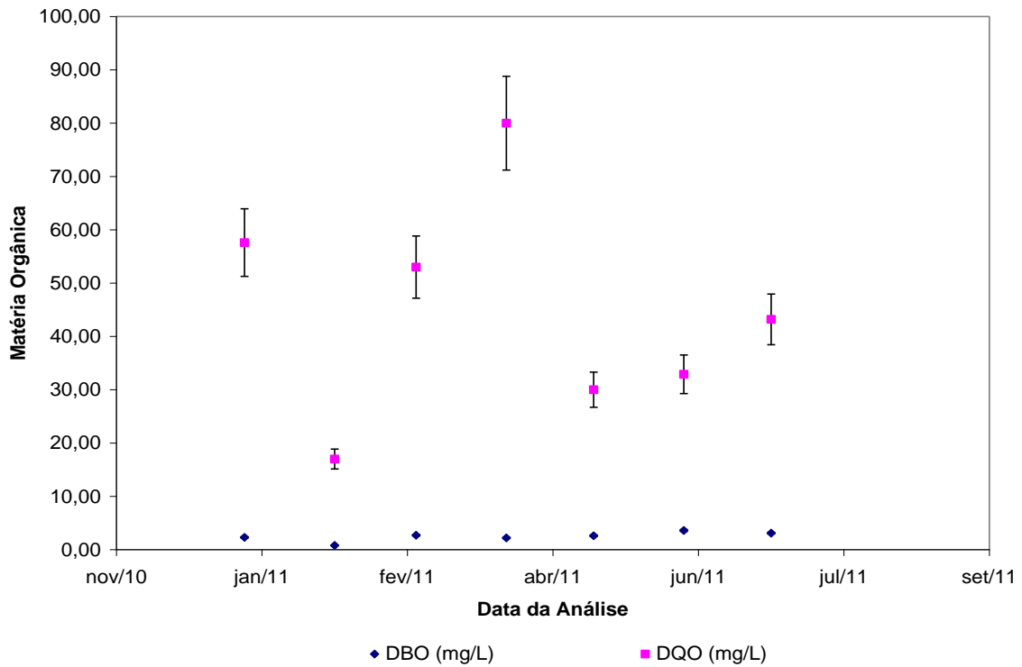
Figura 7: Variações da DBO e DQO na Lagoa de Extremoz-RN.
