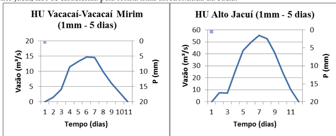
Figura 3 - Hidrogramas Unitários das bacias analisadas.
