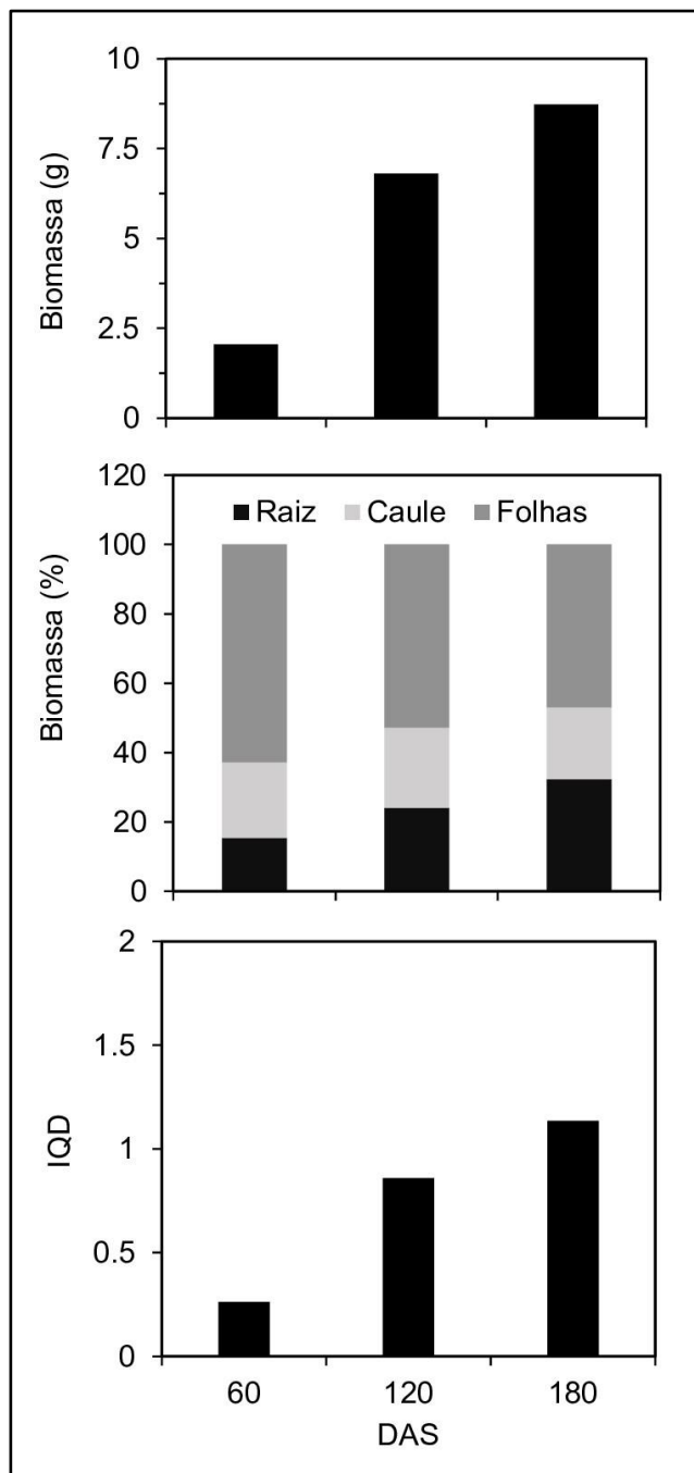
Figura 3 – Biomassa dos compartimentos das mudas (raiz, caule e folha) e índice de qualidade de Dickson (IQD) de Dipteryx alata Vog produzidas a partir de sementes coletadas em Jataí-GO após 60, 120 e 180 dias da semeadura (DAS)
