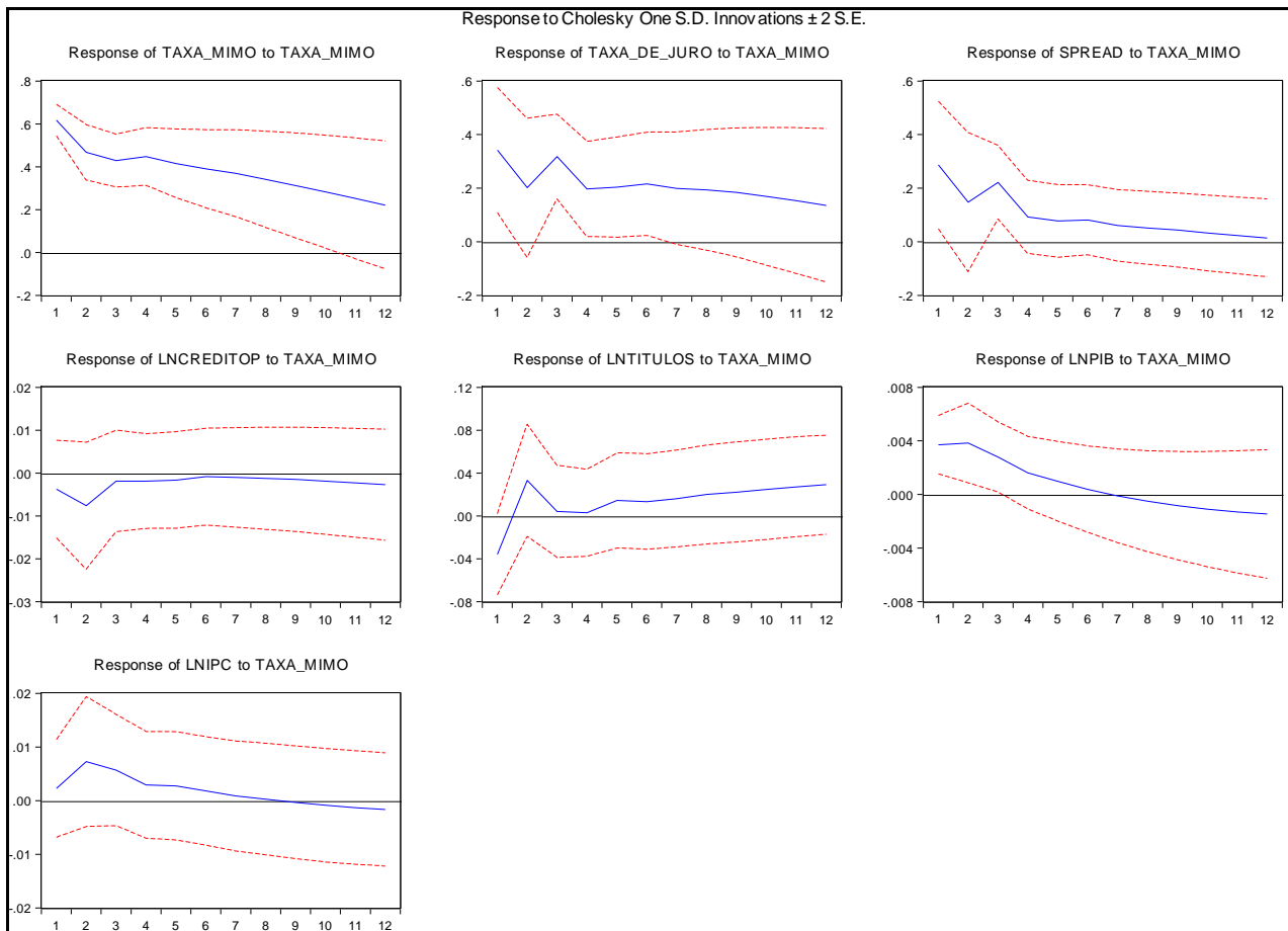
Figura 1 – Função Impulso Resposta
