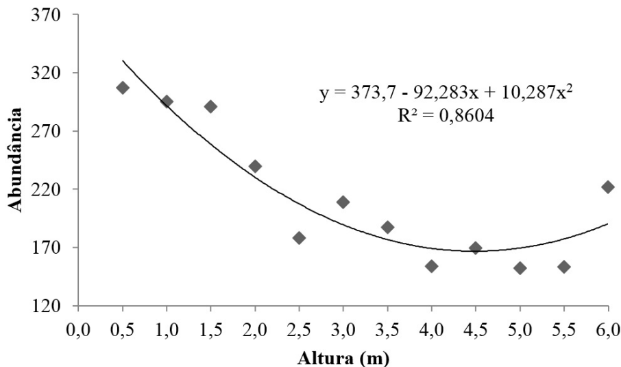
FIGURA 3: Abundância de escolitíneos em diferentes alturas, coletados através de armadilha de interceptação de voo em povoamento de Pinus taeda , no período de 03/11/2011 a 29/05/2012, em Santa Maria - RS.
