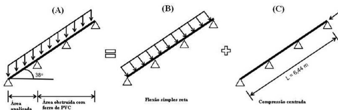
FIGURA 8: Solicitação dos caibros por flexão composta reta (a), ilustrando as componentes transversal (b) e paralela (c) ao eixo longitudinal do caibro.
