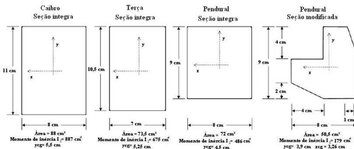
FIGURA 9: Seções transversais da “situação íntegra e da situação modificada”.
