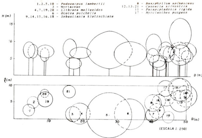
FIGURA 1: Perfil esquemático vertical e horizontal de um trecho do “capão”, para as árvores com DAP > 15 cm.
