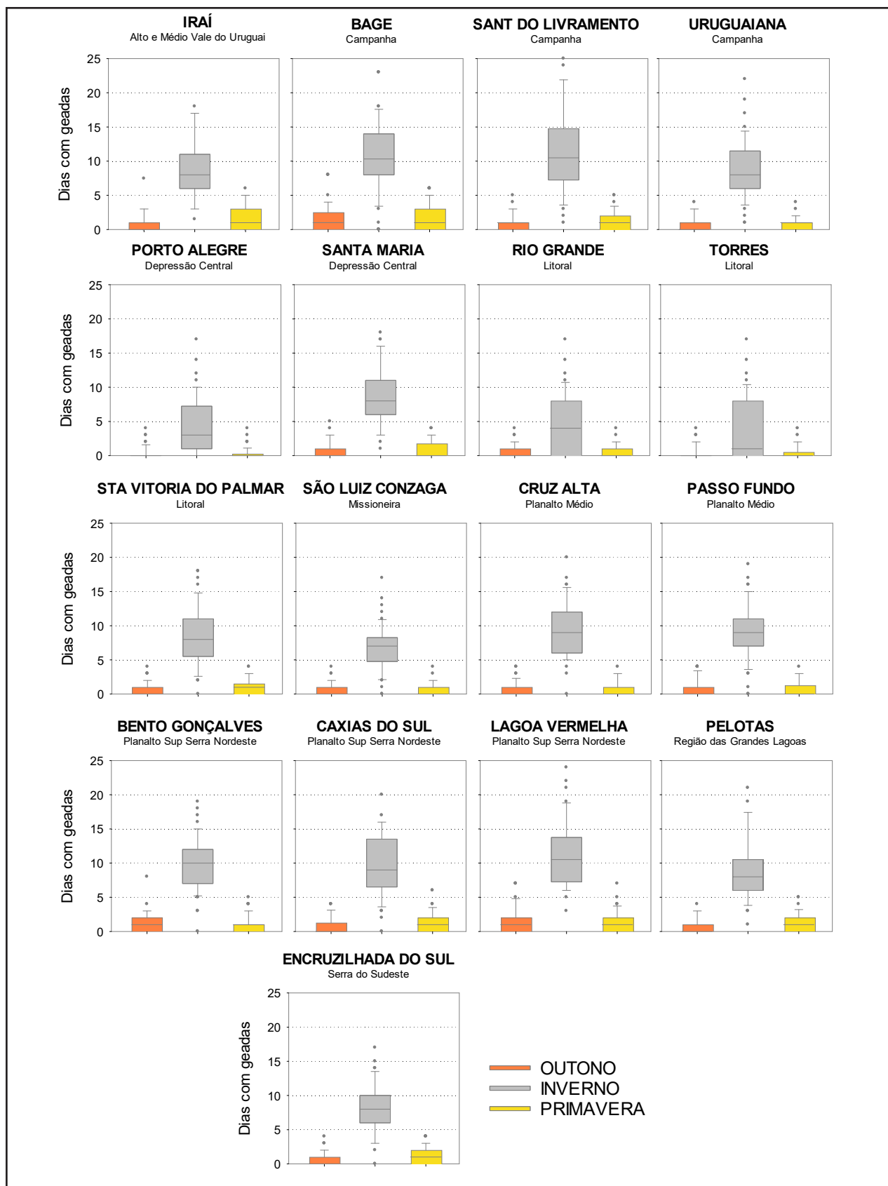
Figura 1 – Diagrama de caixas do número de dias com geada para as estações do outono, inverno e primavera, em diversas localidades do RS. Período: 1961 a 2021
