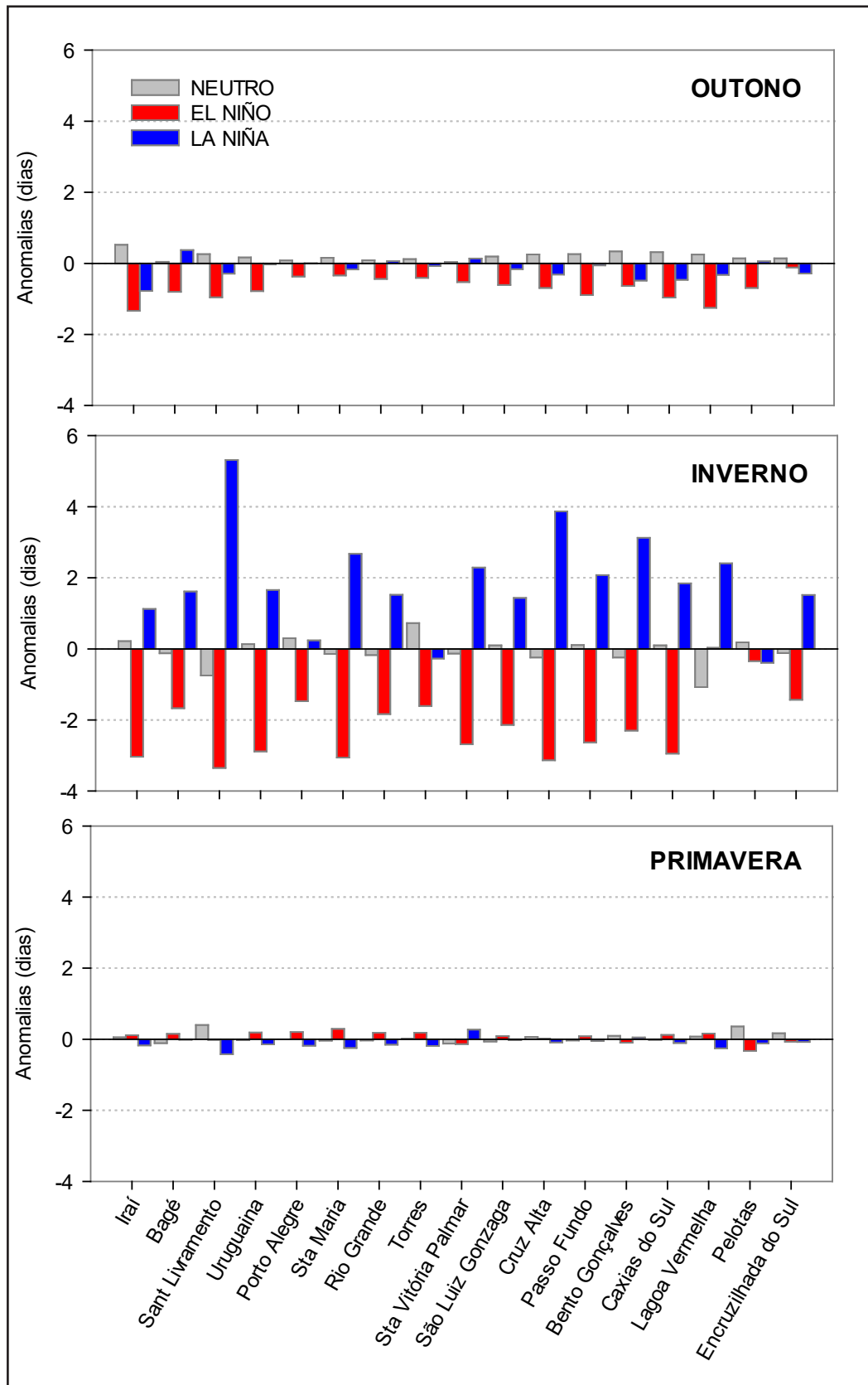
Figura 3 – Anomalias médias do número de dias de geadas associadas a eventos El Niño, La Niña e Neutro, no outono, inverno e primavera, no RS. Período: 1961-2021
