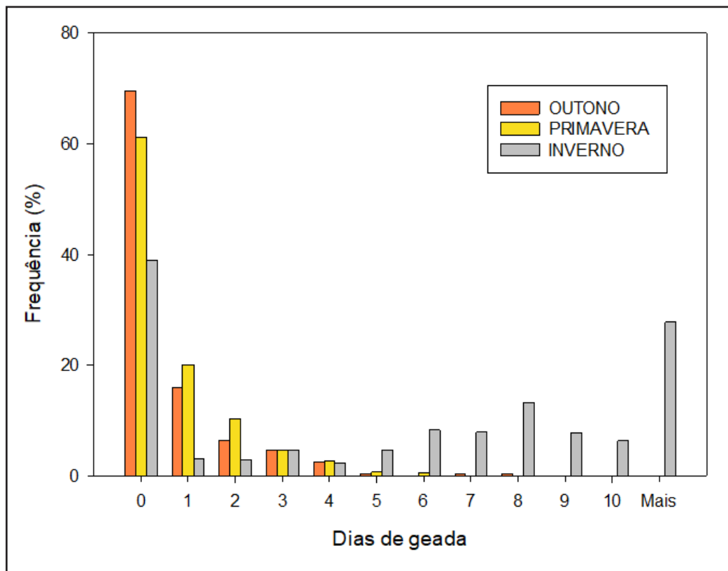
Figura 2 – Histograma de frequência de ocorrência de DG no outono, inverno e primavera, em todo o estado do Rio Grande do Sul, período 1961 a 2021
