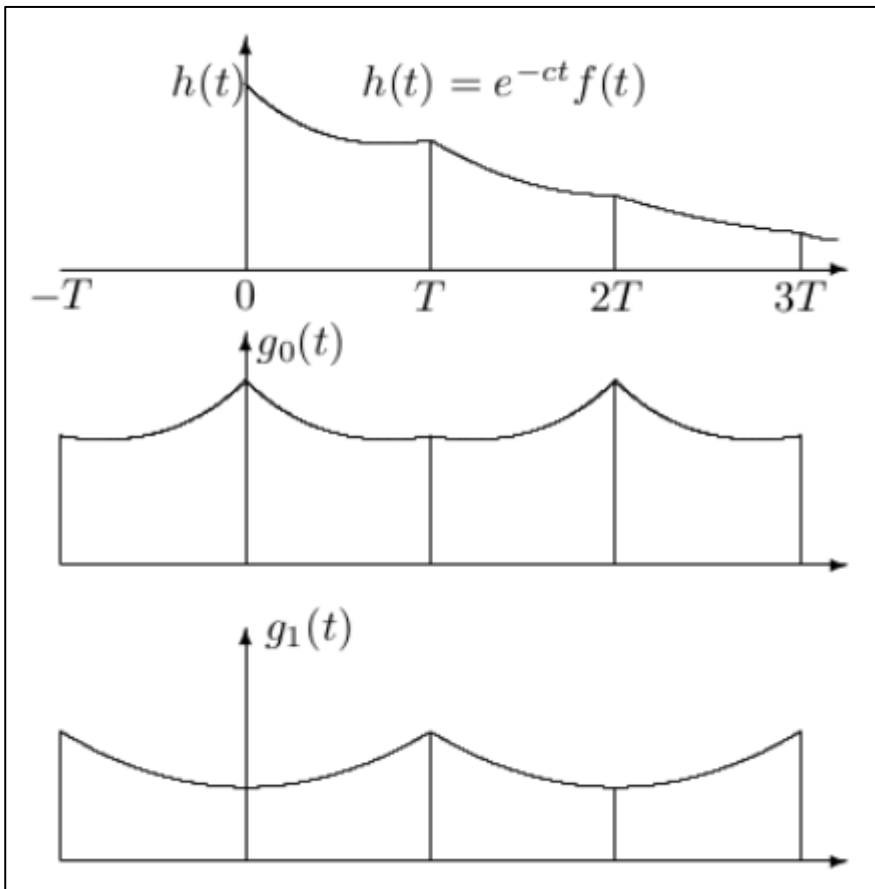
Figura 1 – Funções h(t) e g_h(t) (Cohen, 2007)
