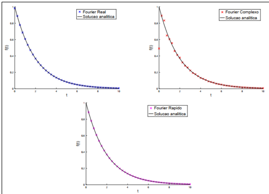
Figura 2 – Comparação dos métodos para inversão de F_7(s) , com a = 0,5 e N = 100
