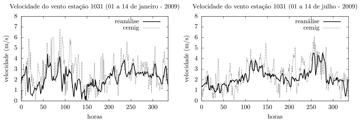
Figura 3: Gráfico comparativo de velocidade do vento para a estação 1031 - Reanálise x Cemig.
