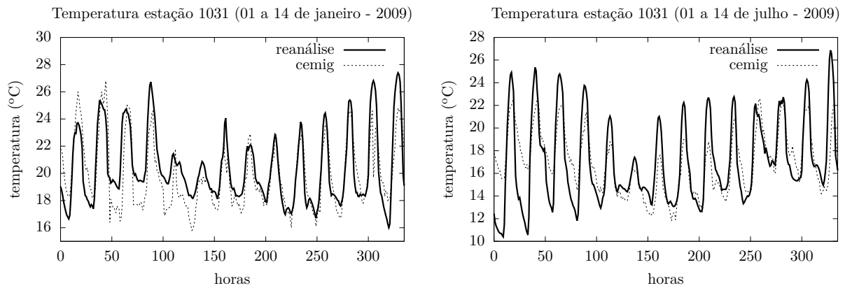
Figura 2: Gráfico comparativo de temperatura para a estação 1031 - Reanálise x Cemig.
