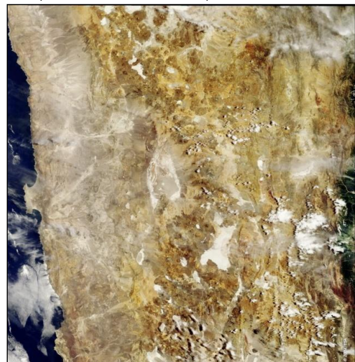
Figura 3 – Deserto de Atacama, visto de imagem de satélite.
