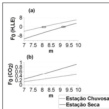
Figura 8 - Funções de otimização do parâmetro m. (a) F 0 (LE,H). (b) F 0 (CO 2 )
