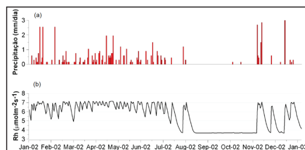
Figura 2 - Médias diárias do ano de 2002 para: (a) precipitação, (em \text{mm}/\text{dia} ). (b) respiração heterotrófica, (em \mu\text{molm}^{-2} \text{s}^{-1} )
