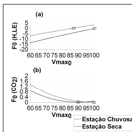
Figura 7 - Funções de otimização do parâmetro Vmax 0 . (a) F 0 (LE,H). (b) F 0 (CO 2 )
