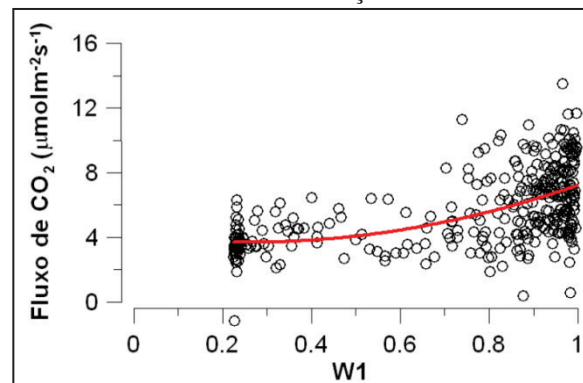
Figura 1- Regressão polinomial entre a média diária noturna de \text{CO}_2 (em \mu\text{molm}^{-2} \text{s}^{-1} ) e a média diária do grau de saturação do solo na primeira camada (em \text{m}^3 \text{m}^{-3} ). Rh = 4,08 - 3,22^* (W1) + 6,35 (W1)^2
