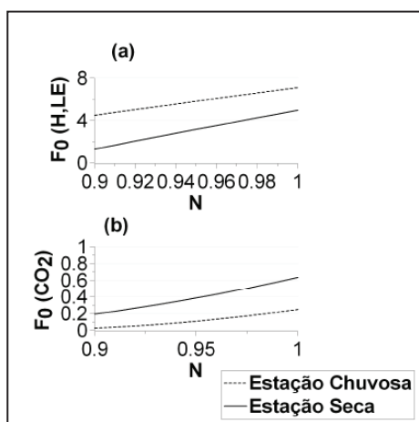
Figura 6 - Funções de otimização do parâmetro N. (a) F 0 (LE,H). (b) F 0 (CO 2 )
