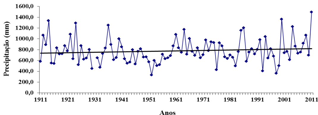
Figura 3 - Análise da tendência pelo teste de Mann Kendall na série temporal de precipitação para os anos de 1911 a 2011 de Campina Grande –PB (Fonte: UACA/UFCEG)
