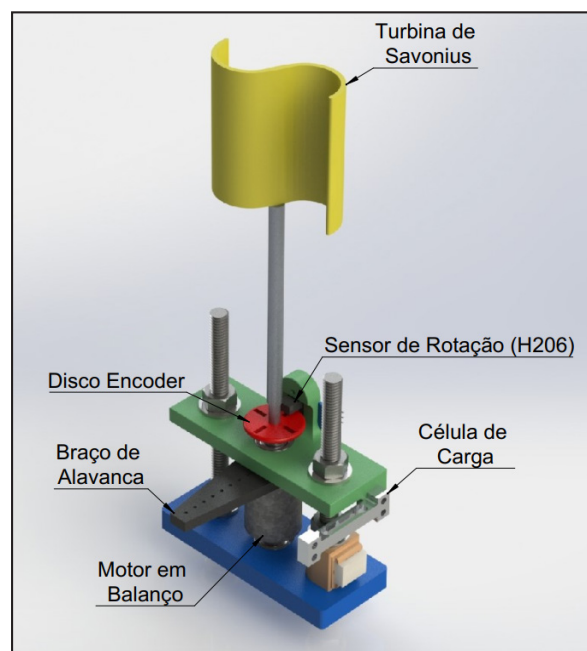
Figura 1 – Dinamômetro proposto
